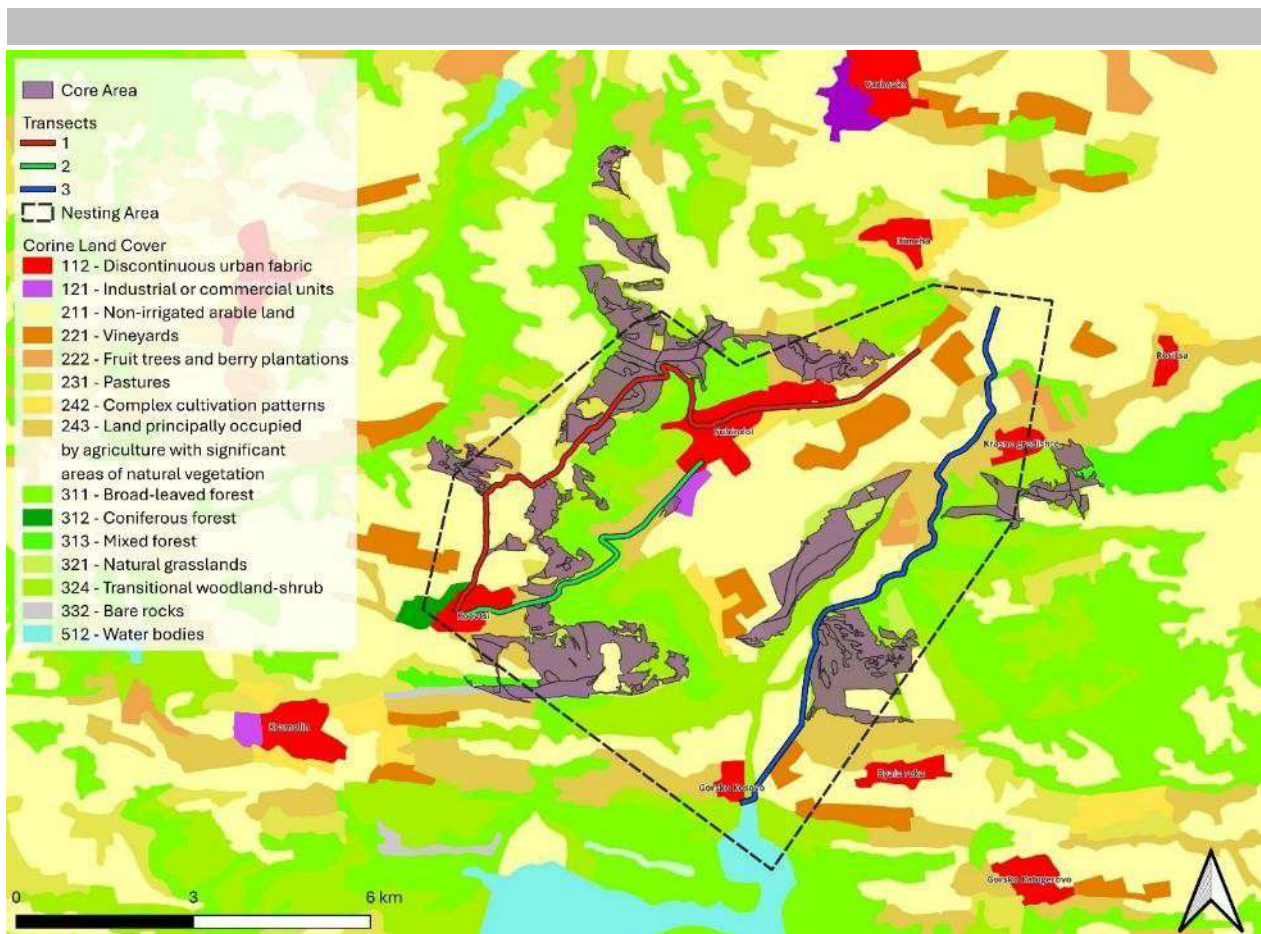
Фигура 49 Типове земно покритие по данни от Корине земно покритие 2018
