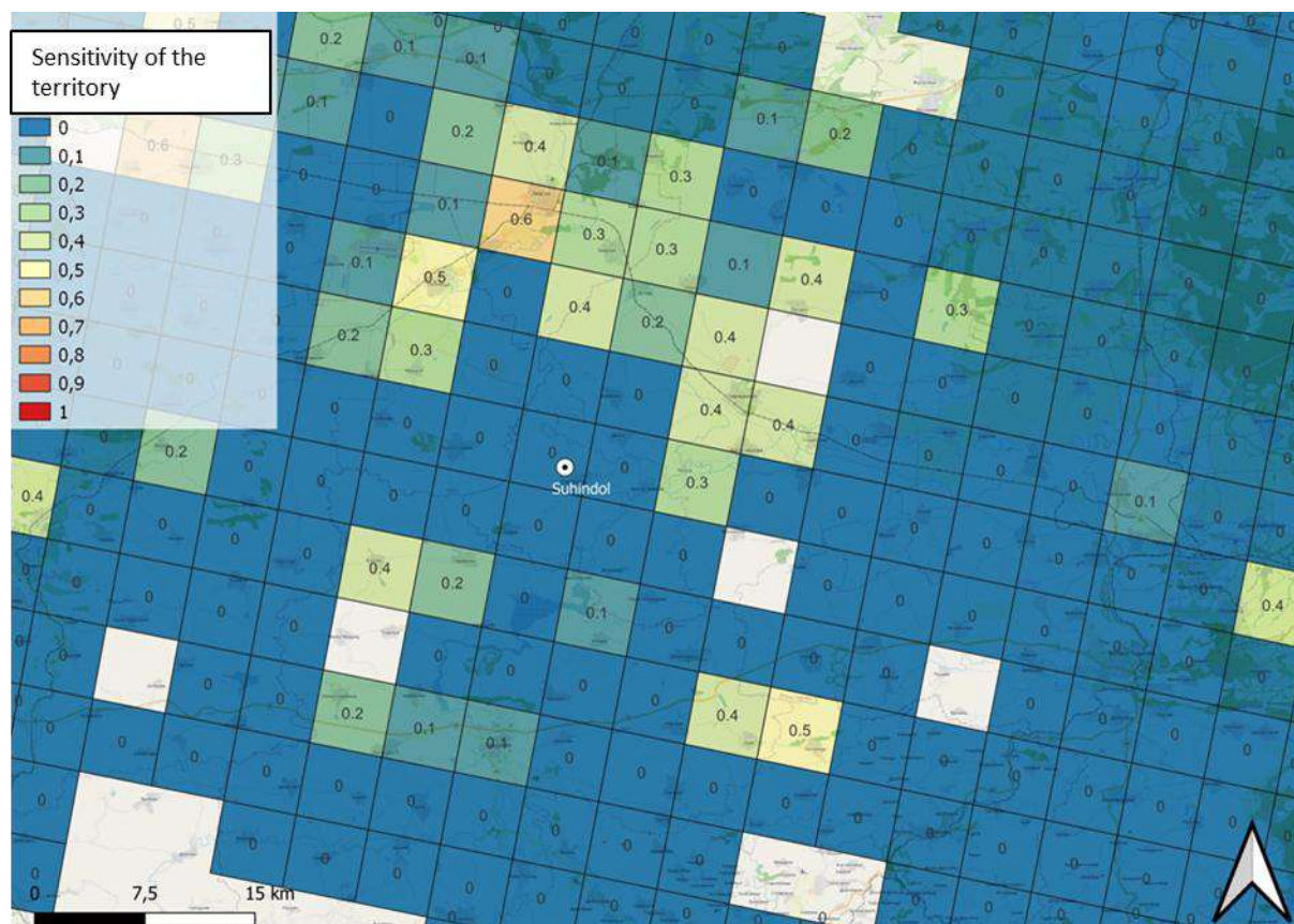
Фигура 20 Оценка на чувствителността на изследваната територия според публикувано изследване. Hotspots in the grid: Avian sensitivity and vulnerability to collision risk from energy infrastructure interactions in Europe and North Africa
