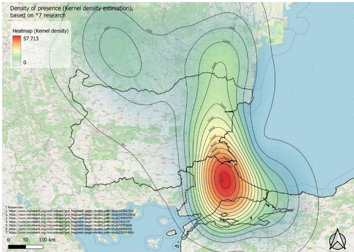
Фигура 60 Разположение на Община Сухиндол по отношение на установените концентрации на мигриращи реещи се птици, през пролетта, по данни от 12 независими проучвания чрез GPS проследяване през територията на България по данни от Макс Планк Институт, Германия ( https://www.movebank.org/cms/movebank-main )
