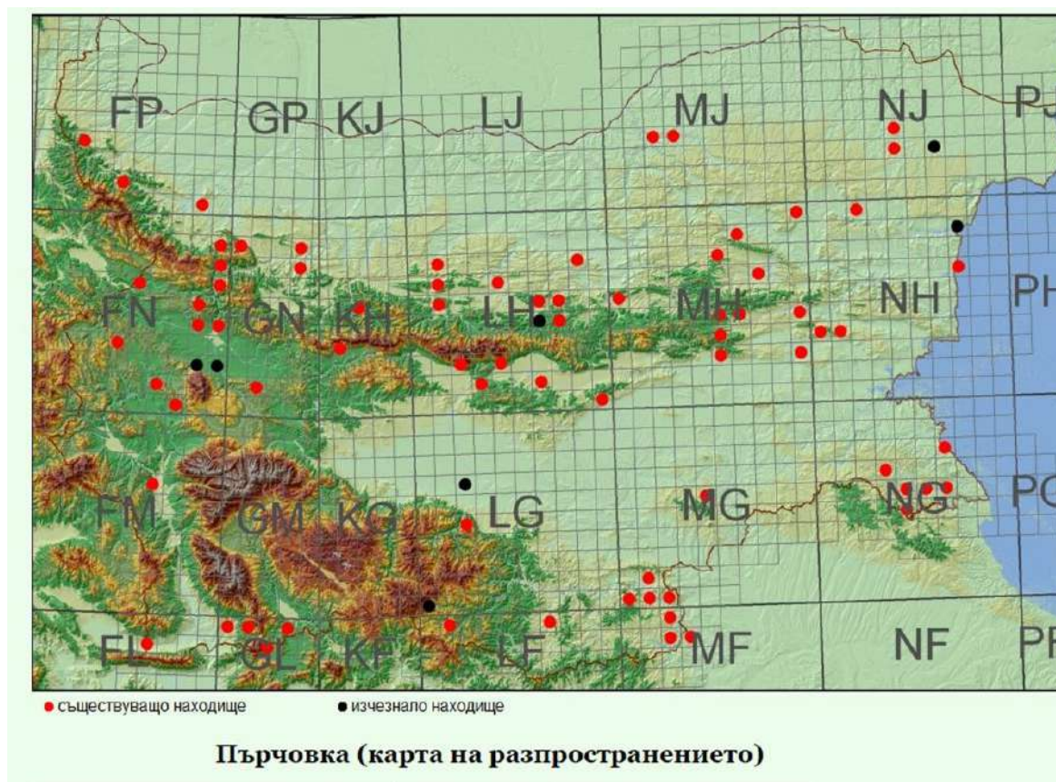
Фигура 41 Карта на разпространение на вида обикновена пърчовка, Himantoglossum caprinum . Източник: Червена книга на Р. България, том I Растения
