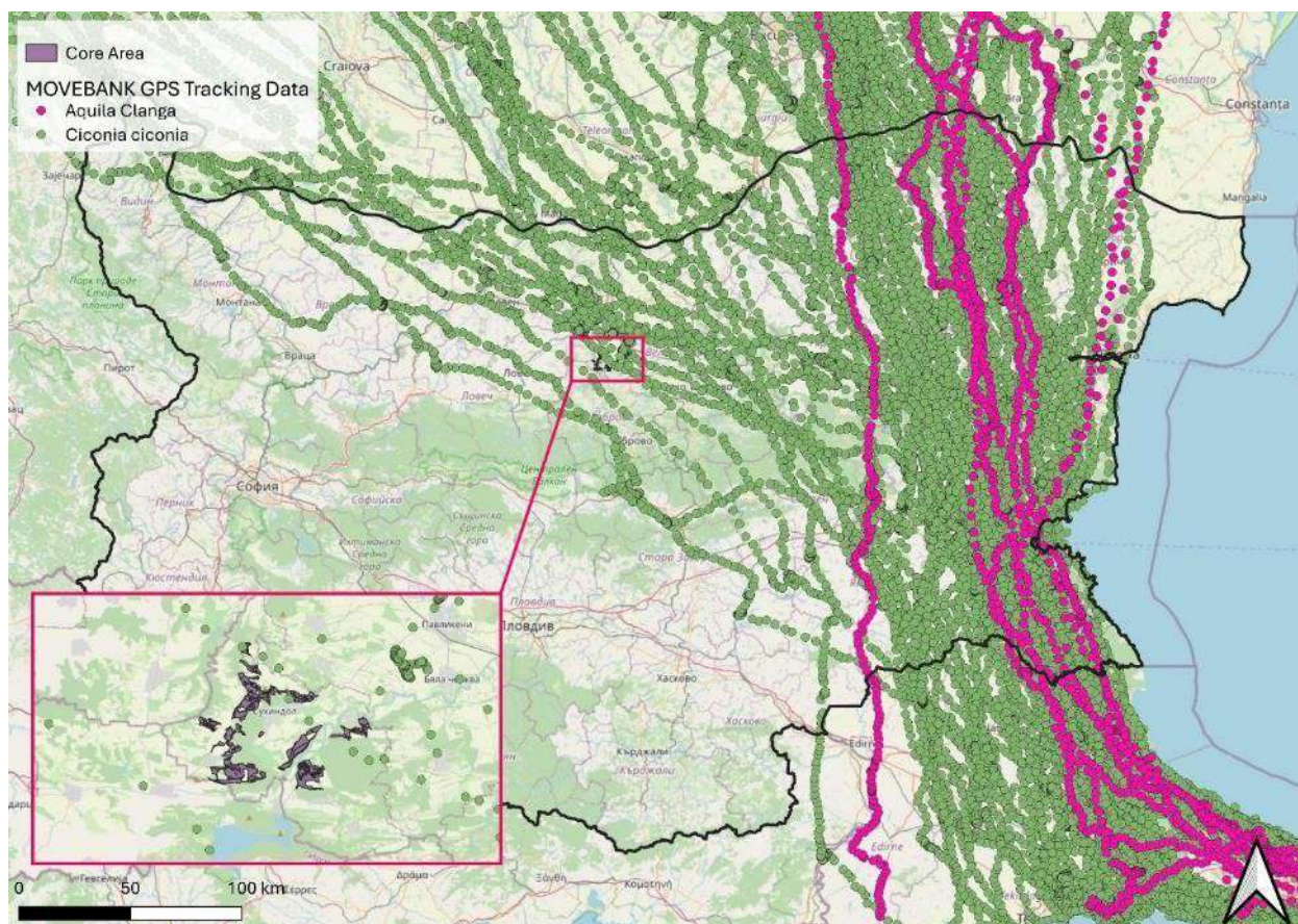
Фигура 59 Извадка от използваните данни от GPS проследяване на реещи се птици използвани при ГИС анализа на територията на община Сухиндол и мигриращите през пролетта птици. (данни от Макс Планк Институт, Германия ( https://www.movebank.org/cms/movebank-main ))
