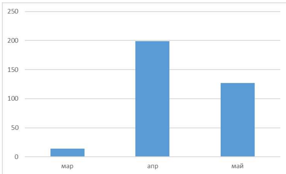
Фигура 57 Динамика на прелета на реещите се видове птици по месеци през пролетния сезон на миграция установени чрез визуални наблюдения в територията.
