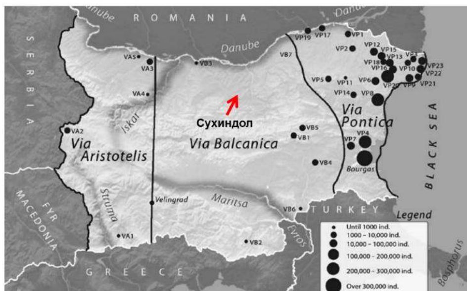
Фигура 53 Общ брой на реещите птици по време на есенната миграция в 35 точки през периода 2004 – 2011 г. (по Tanyo M. Michev, Lyubomir A. Profirov, Nikolay P. Karaivanov, Boyan T. Michev 2012. Migration of Soaring Birds over Bulgaria Acta zool. bulg., 64 (1),: 33-41) и разположението на община Сухиндол.
