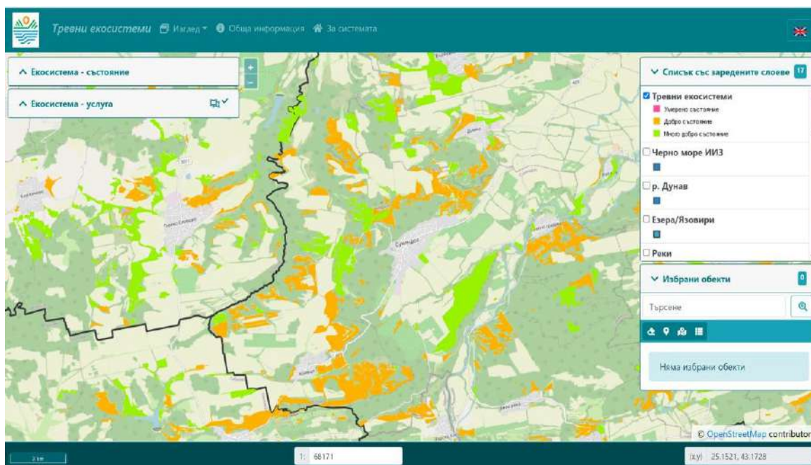
Фигура 24 Данни в базата на ИАОС за състояние на екосистемите на тревните съобщества. Източник: ( https://ecosys.eea.government.bg/grasslands/ ).
