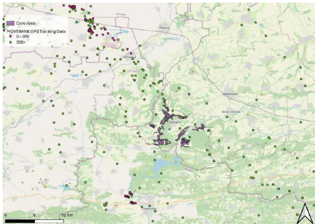
Фигура 25 Извадка от GPS проследяване в радиус от 30 км около територията използвани при ГИС анализа на височината на прелета (данни от Макс Планк Институт, Германия ( https://www.movebank.org/cms/movebank-main ))
