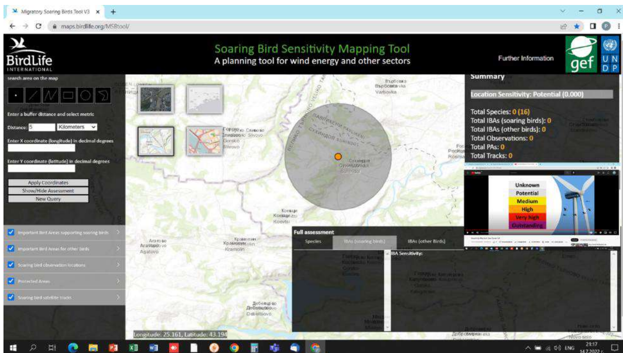
Фигура 19 Оценка на чувствителността на изследваната територия според специално създаден от BirdLife International интернет инструмент за оценка на риска от БЕИ за птиците ( https://maps.birdlife.org/MSBtool/ ).
