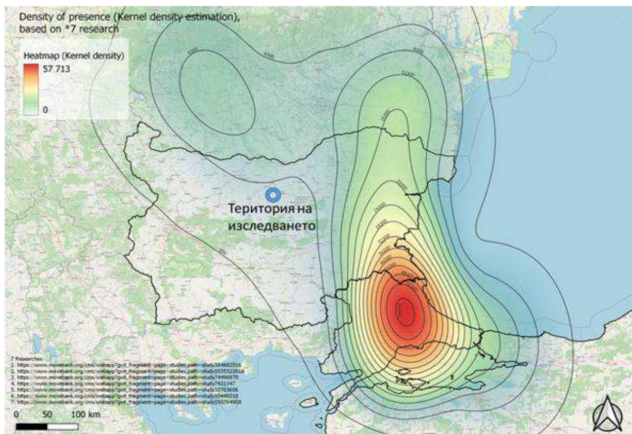
Фигура 21 Разположение на изследваната територия по отношение на установените чрез проследяване с GPS (Global Positioning System) мигриращи бели щъркели (по данни от Макс Планк Институт : https://www.movebank.org/cms/movebank-main )
