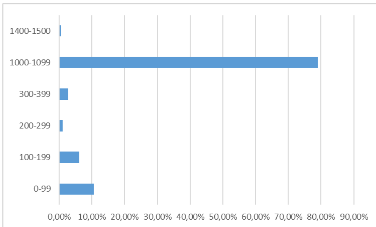
Фигура 56 Височинно разпределение на установените през есента мигриращи птици през изследваната територия (на община Сухиндол)
