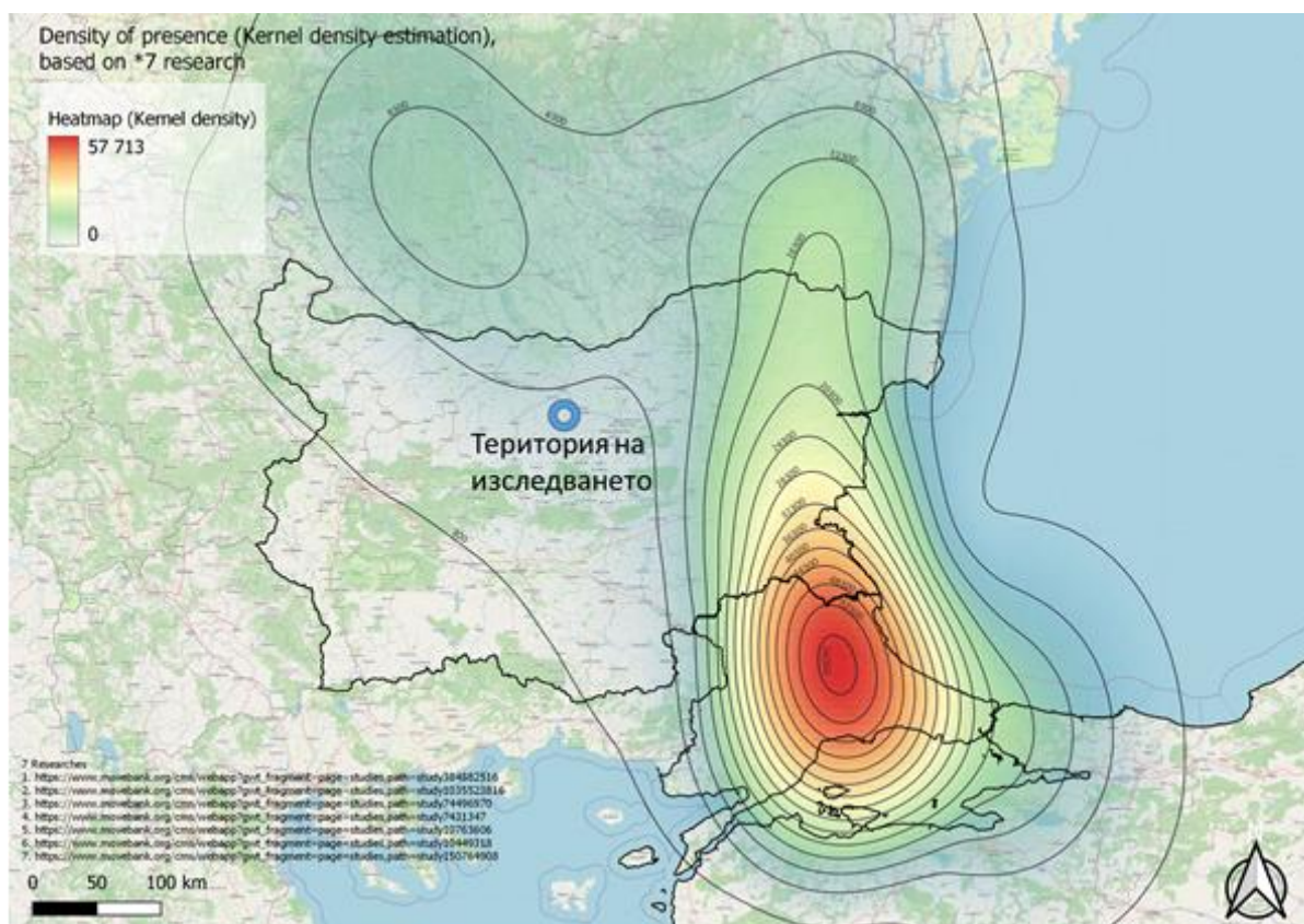
Фигура 51 Разположение на изследваната територия по отношение на установените чрез проследяване с GPS (Global Positioning System) мигриращи бели щъркели (по данни от Макс Планк Институт : https://www.movebank.org/cms/movebank-main )
