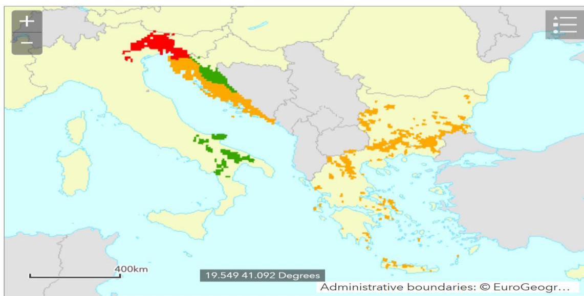
Фигура 30 Разпространение и природозащитно състояние на местообитание 62A0 в Европа (Източник: EUNIS -Factsheet for Eastern sub-mediterranean dry grasslands (Scorzoneralia villosae) ).
