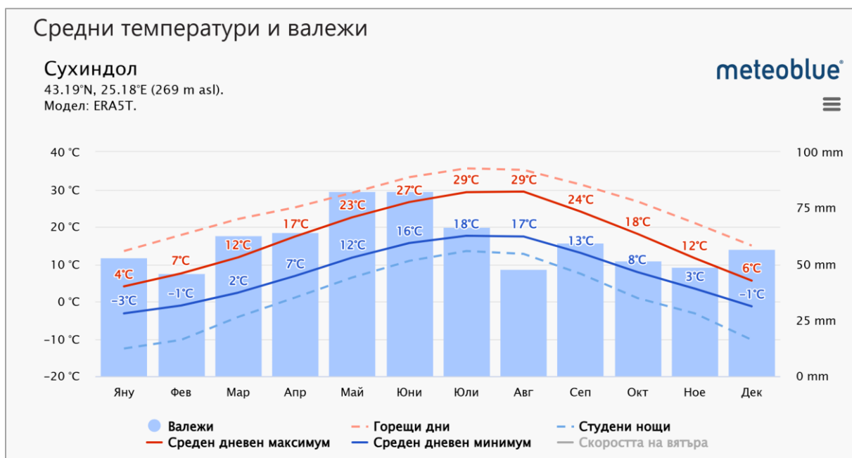
Фигура 14 Средни температури и валежи в района на община Сухиндол. Източник: Симулативни исторически данни за климата и времето за Сухиндол - meteoblue
