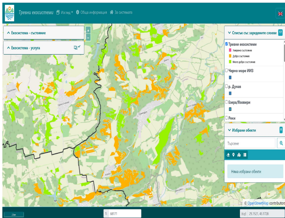
Фигура 24 Данни в базата на ИАОС за състояние на екосистемите на тревните съобщества. Източник: ( https://ecosys.eea.government.bg/grasslands/ ).
