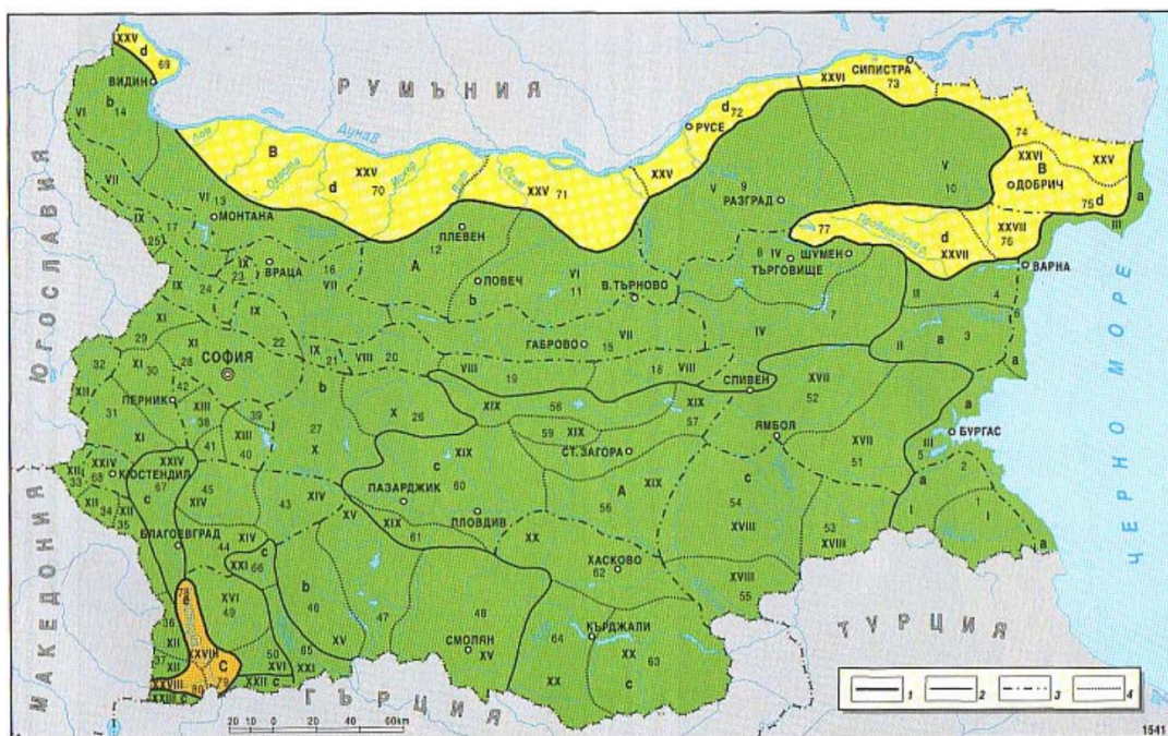
Фигура 23 Геоботаническо райониране на България (по Бондев, 1997)
