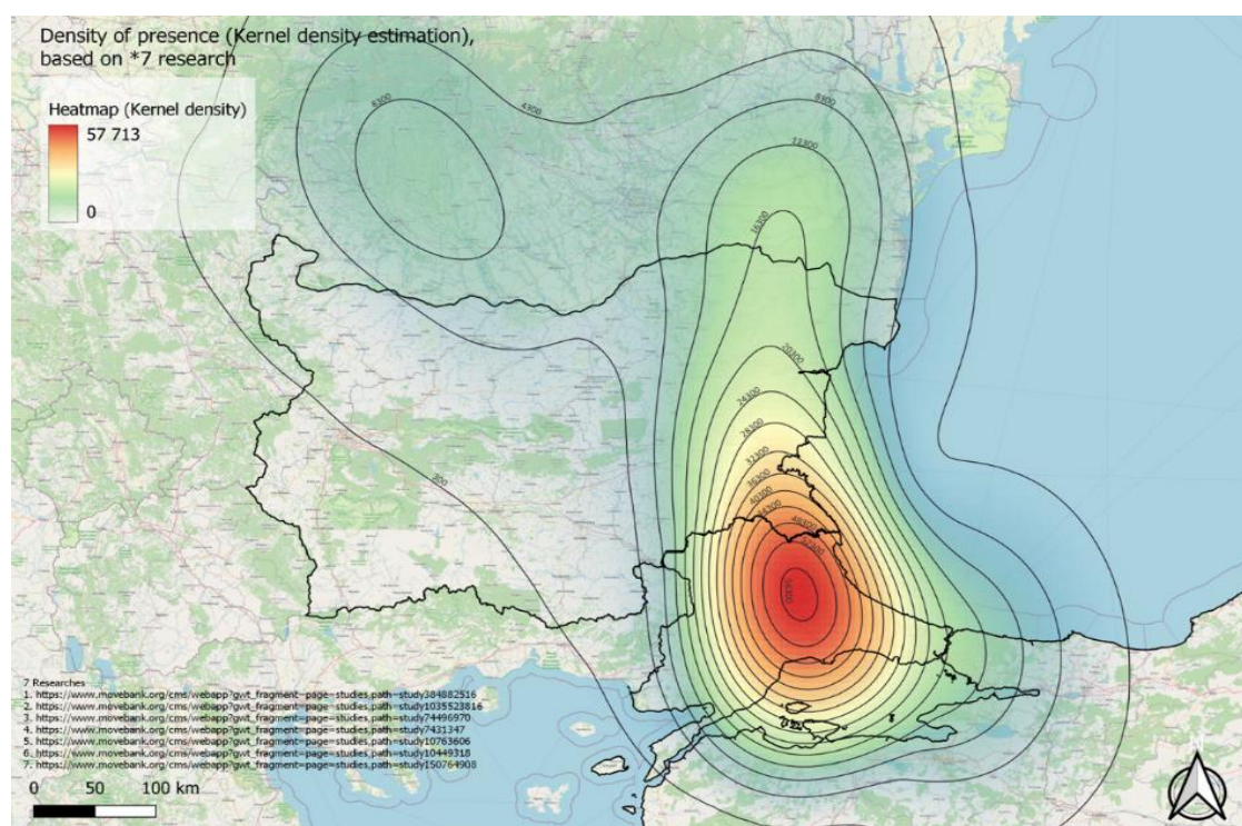
Фигура 59 Извадка от използваните данни от GPS проследяване на реещи се птици използвани при ГИС анализа на територията на община Сухиндол и мигриращите през пролетта птици.(данни от Макс Планк Институт, Германия ( https://www.movebank.org/cms/movebank-main ))
