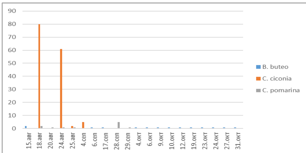
Фигура 52 Интензивност на есенната мигрирцията на трите най-многочислени вида птици: обикновен мишелов (синьо), малък креслив орел (сиво) и бял щъркел (червено) над територията на община Сухиндол (данни визуални наблюдения есен 2022 г.
