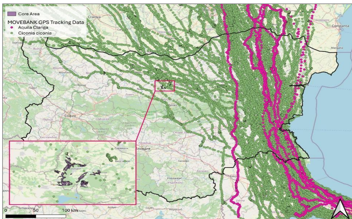
Фигура 59 Извадка от използваните данни от GPS проследяване на реещи се птици използвани при ГИС анализа на територията на община Сухиндол и мигриращите през пролетта птици.(данни от Макс Планк Институт, Германия ( https://www.movebank.org/cms/movebank-main ))
