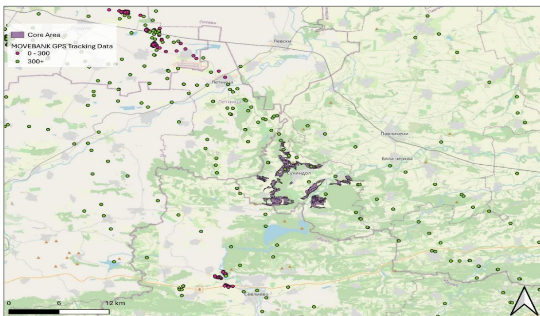
Фигура 61 Извадка от GPS проследяване в радиус от 30 км около територията използвани при ГИС анализа на височината на прелета (данни от Макс Планк Институт, Германия ( https://www.movebank.org/cms/movebank-main ))
