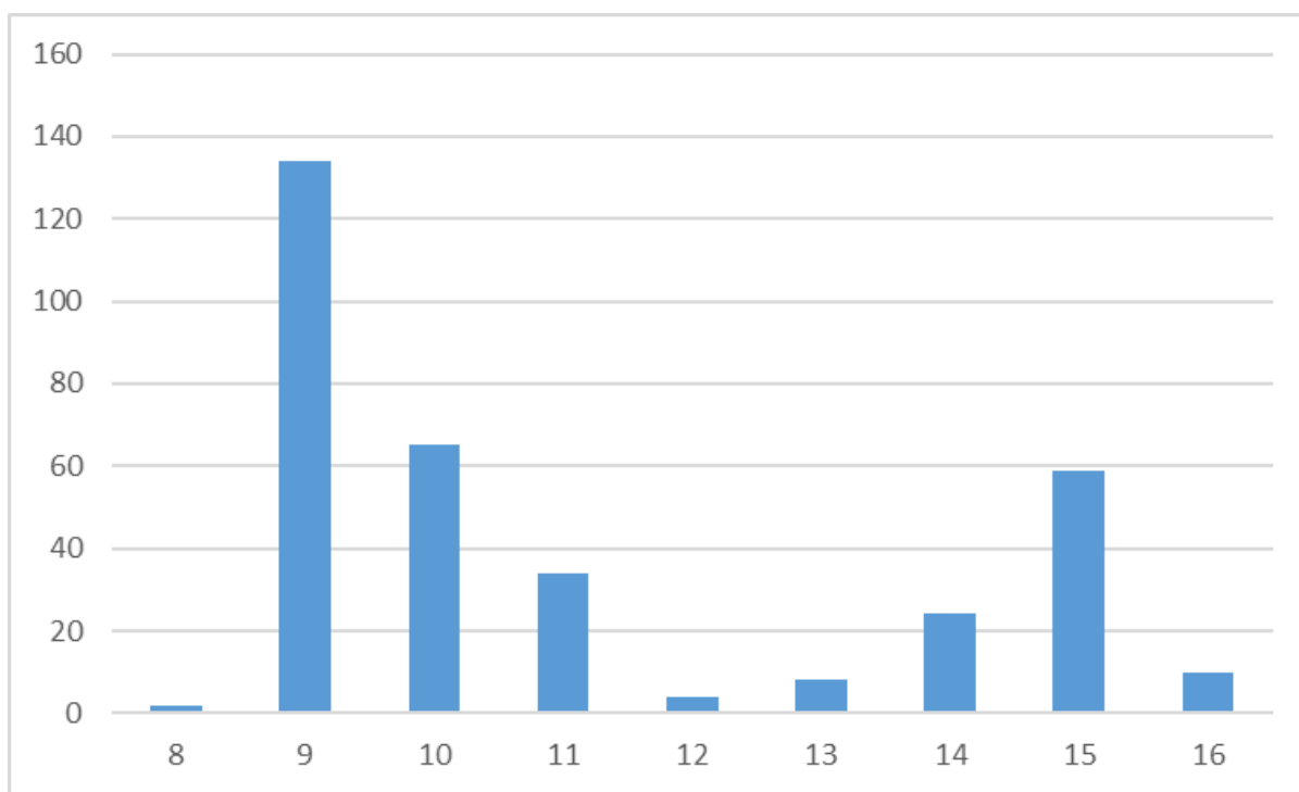
Фигура 58 Часова динамика на мигриращите реещи се птици от всички видове през територията на Община Сухиндол (данни визуални наблюдения пролет 2023 г.).
