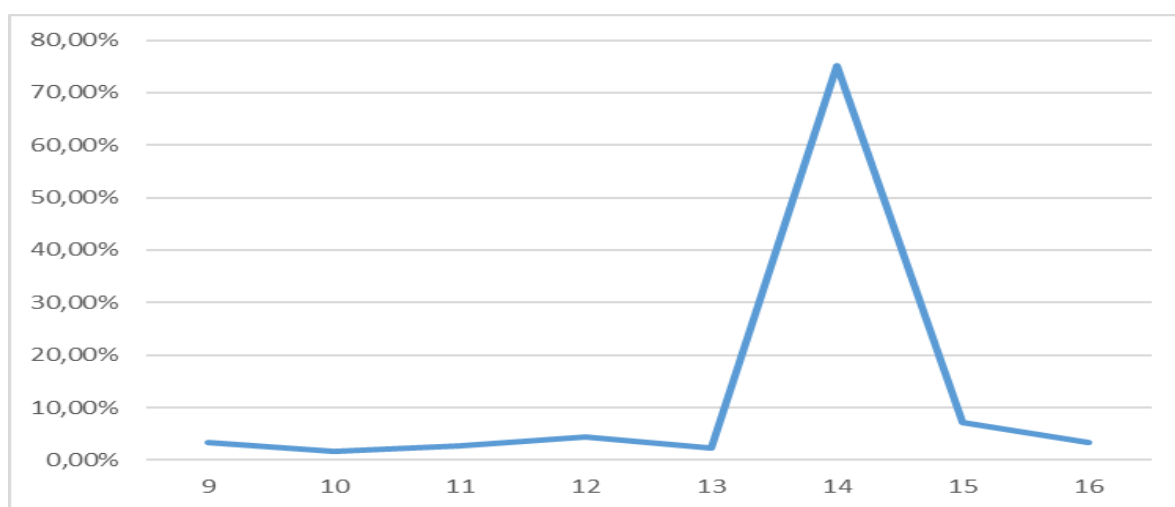
Фигура 12 Часова динамика на мигриращите реещи се птици през територията на община Сухиндол (данни визуални наблюдения есен 2022 г.).
