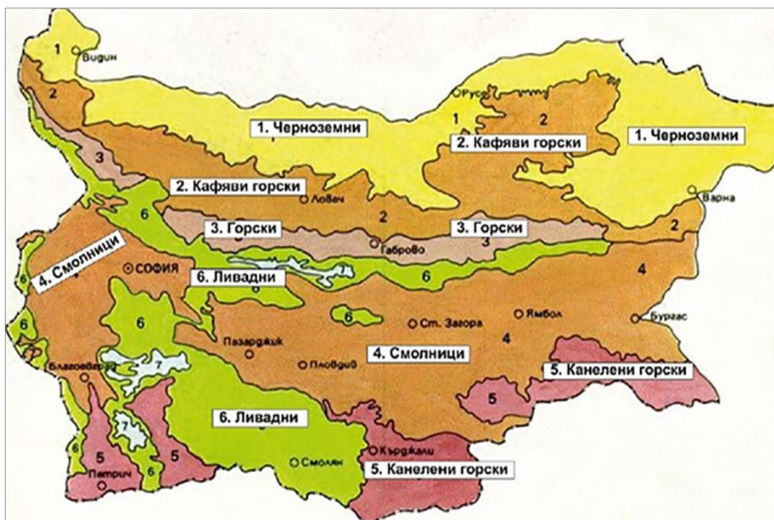
Фигура 18 Почвено-географски райониране на територията на Република България, Атлас на почвите в България
