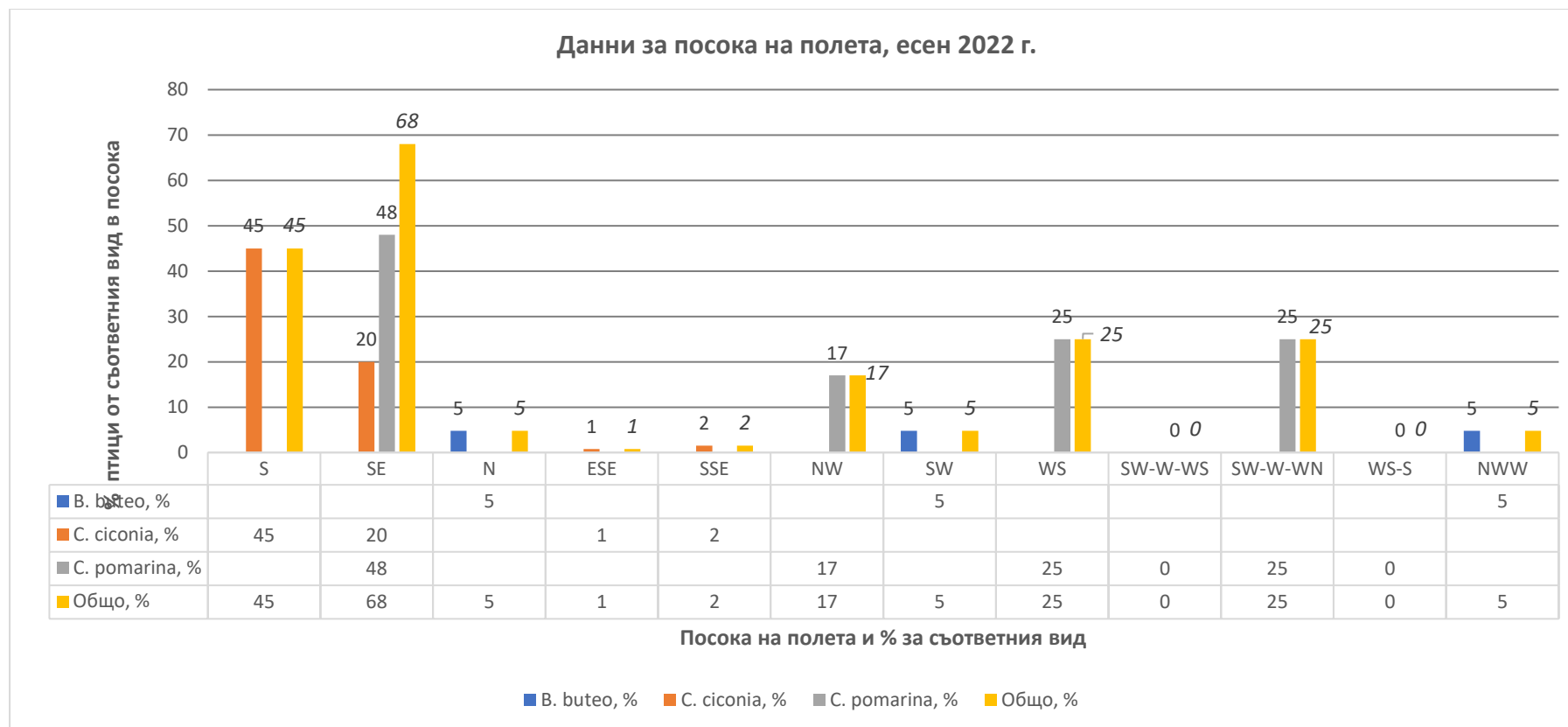
Фигура 54 Посоки на полета на мигриращите реещи се птици през есента по данни от визуални наблюдения през есента на 2022г.
