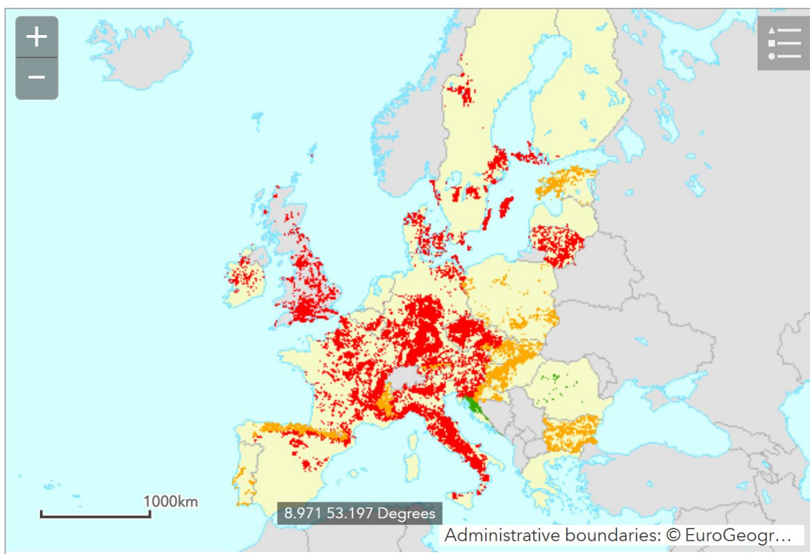
Фигура 37 Разпространение и природозащитно състояние на местообитание 6210 в Европа (Източник: EUNIS -Factsheet for Semi-natural dry grasslands and scrubland facies on calcareous substrates (Festuco-Brometalia) (* important orchid sites).
