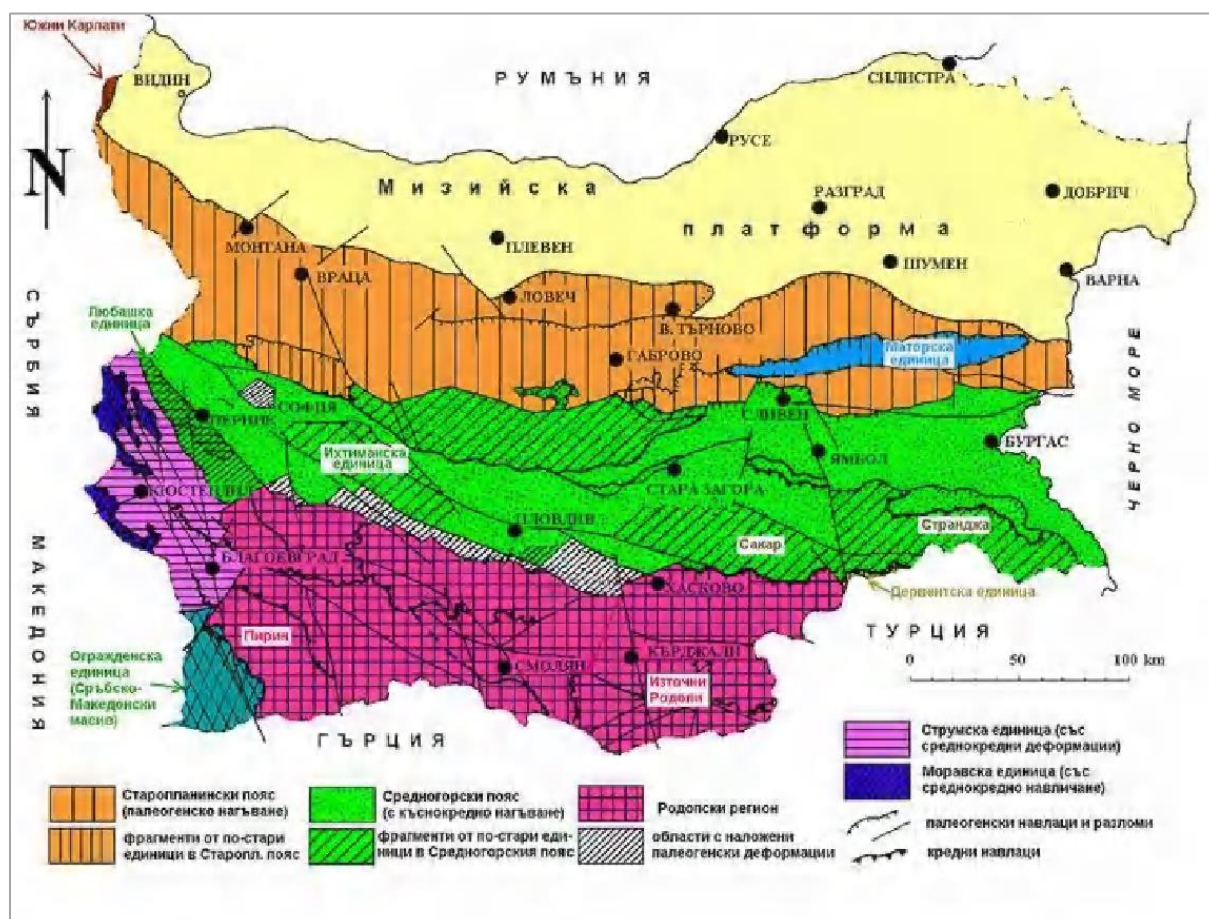
Фигура 15 Геолого-тектонска карта на Република България
