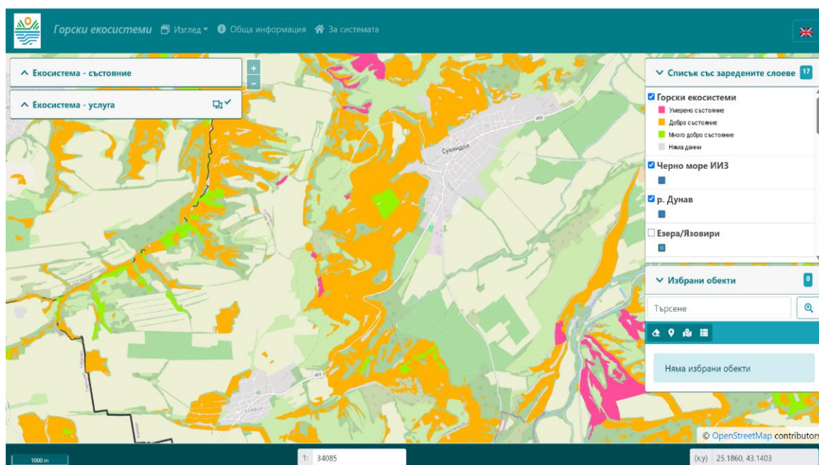
Фигура 38 Данни в базата на ИАОС от картиране на горските екосистеми и техните екосистемни услуги, Източник: ИАОС https://ecosys.eea.government.bg/forest/ .
