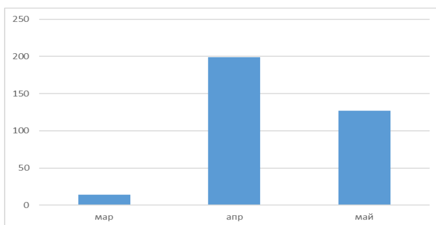
Фигура 57 Динамика на прелета на реещите се видове птици по месеци през пролетния сезон на миграция установени чрез визуални наблюдения в територията.
